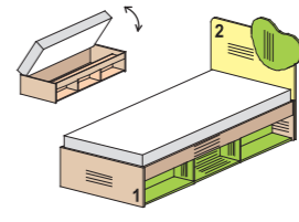
51K013 без матраца 51K014 с матрацем 2064x959x895
