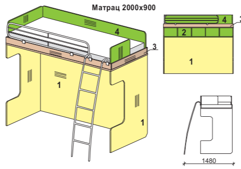
Кровати 51K031 без матраца с лестницей 51K032 с матрацем с лестницей 2086x1480x1773
